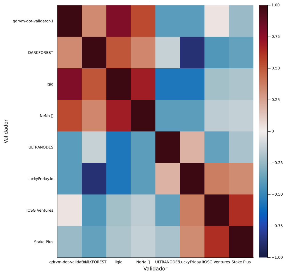
Matriz de Correlação entre Validadores
